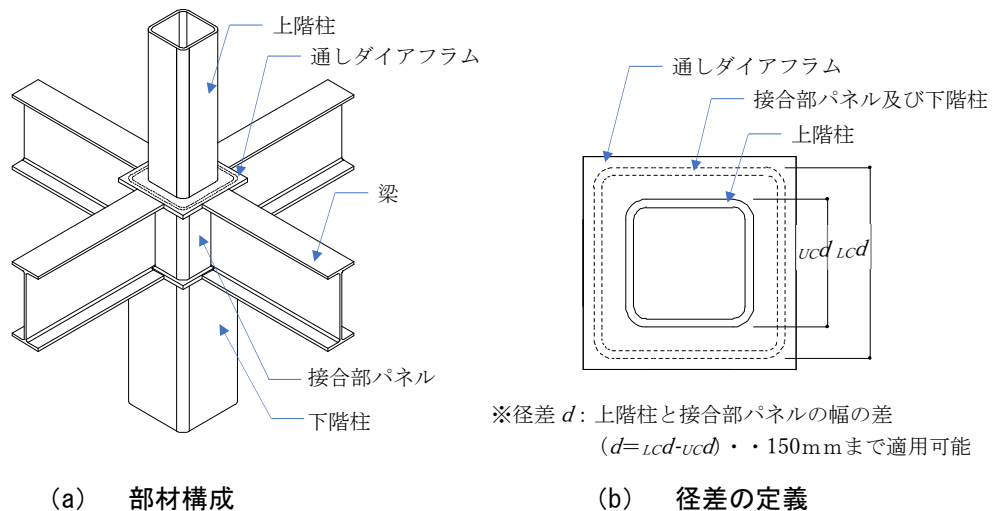
図-2 異幅柱接合部工法の概要
