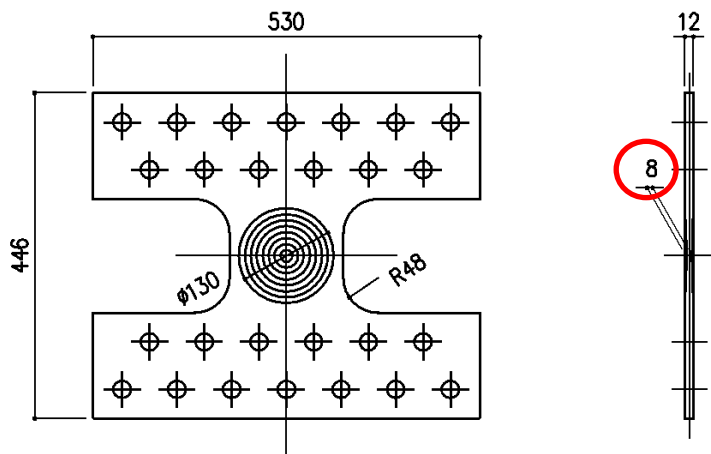
図1 FMS 合金 LSPD の形状
