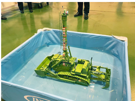
水陸両用ブルドーザのラジコン模型
