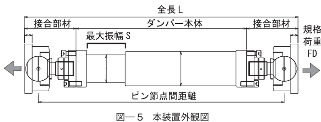
図-5 本装置外観図
