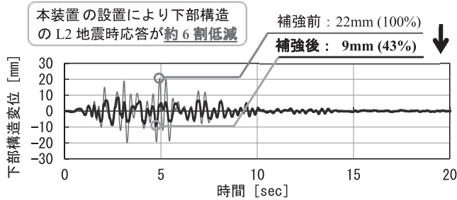
図-7 大規模振動台実験の結果の一例 (レベル2地震動II-II入力時)
