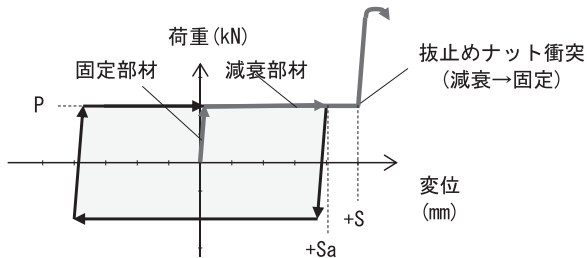
図一 3 本装置の荷重－変位関係
