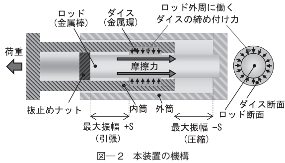
図一 本装置の機構
